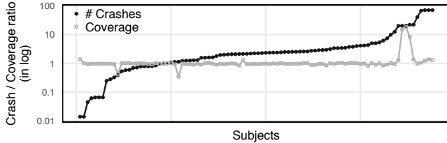
(a) Ankou vs. AFL.
