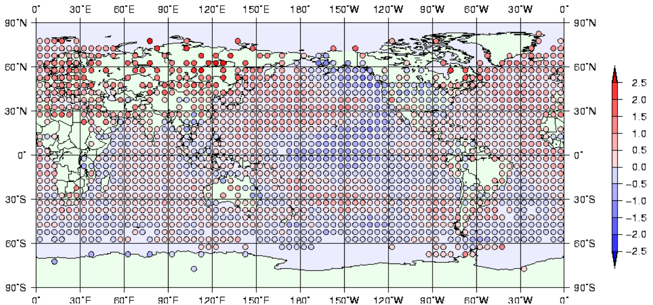
図2 2008年の年平均気温平年差(1～11月)の分布図 各観測点の平年差を緯度、経度5度の領域ごと平均した値で示す。 2008年は、東南アジア、米国、オーストラリア東部を除く陸域のほぼ全域で気温が平年よりも高く、特にユーラシア大陸の中高緯度の陸域では昨年に続き平年よりも高温だった。海面水温は、中部太平洋赤道域から北米大陸西岸にかけての負偏差、西部太平洋赤道域から日本東方海域の正偏差が顕著であった。また、北大西洋高緯度では海面水温が平年より高い状態が続いている。 なお、1891年以降の各月の月平均気温平年差および各年の年平均気温平年差の分布図を次のページに掲載している。
