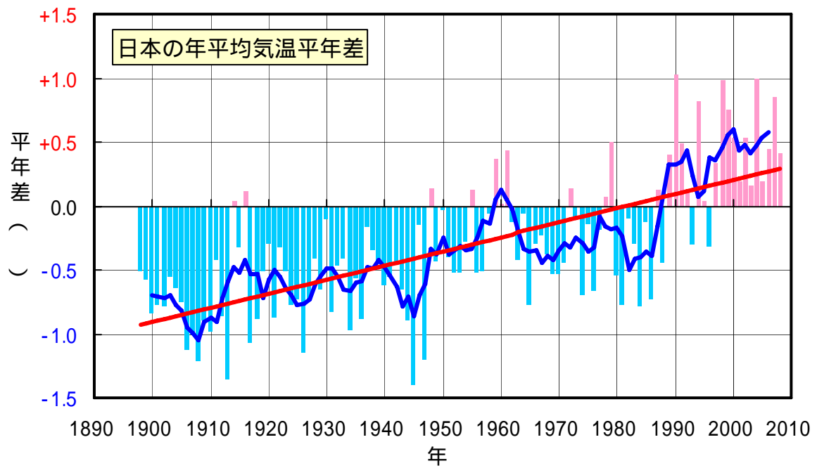
図3 日本の年平均気温の平年差の経年変化(1898～2008年) 棒グラフは各年の値、紺の曲線は各年の値の5年移動平均、赤の直線は長期変化傾向を示す。 ただし、2008年は1月～11月の期間から算出した値(速報値)を用いている。
