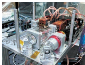
Qswパルスレーザ (与圧筐体封入前の振動試験モデル)
