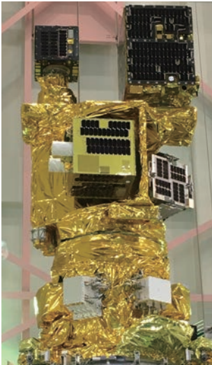
複数衛星搭載構造 [革新的衛星技術実証2号機]
