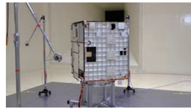
小型実証衛星4号機 (RAISE-4) エンジニアリングモデル
