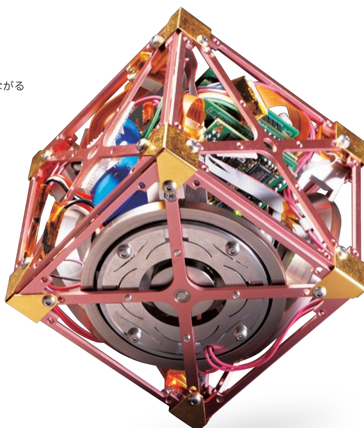
超小型三軸姿勢制御モジュール
