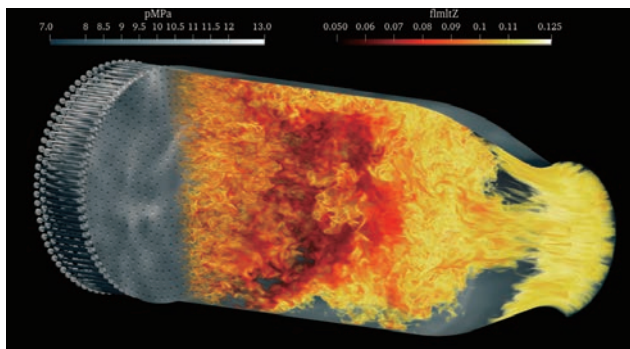
[ロケットエンジン燃焼器] 数値シミュレーション
