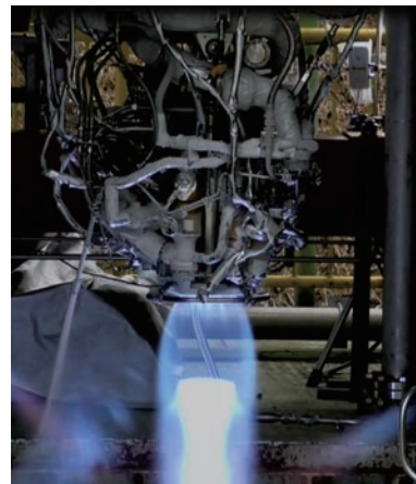
推力30kN高性能メタンエンジン試作品の燃焼試験
