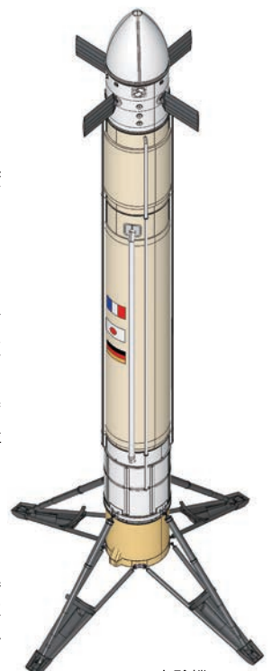
CALLISTO実験機の 着陸時の形態
