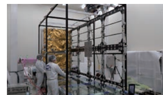
展開型軽量パネルの展開試験
