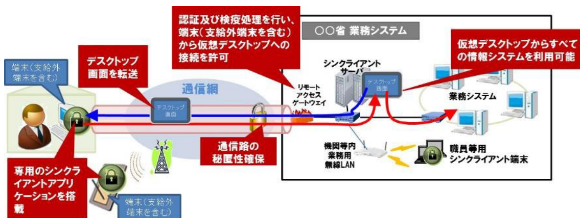
図 7.1.1-1 シンクライアントのシステム構成例
