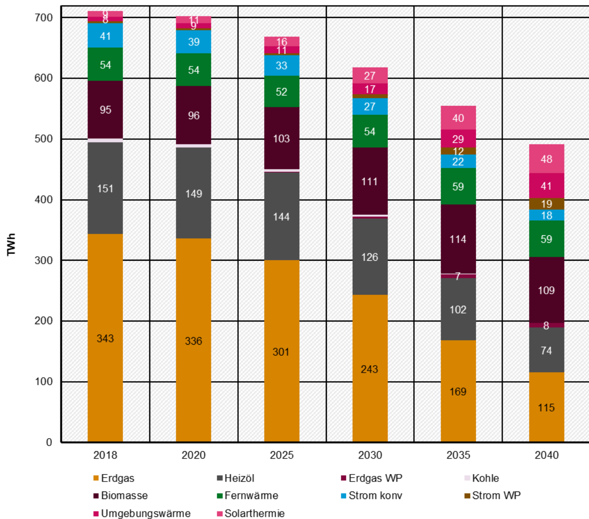
Abbildung 31: Entwicklung des Endenergiebedarfs für Raumwärme und Warmwasser in Wohngebäuden und Nichtwohngebäuden (GHD) im MMS
