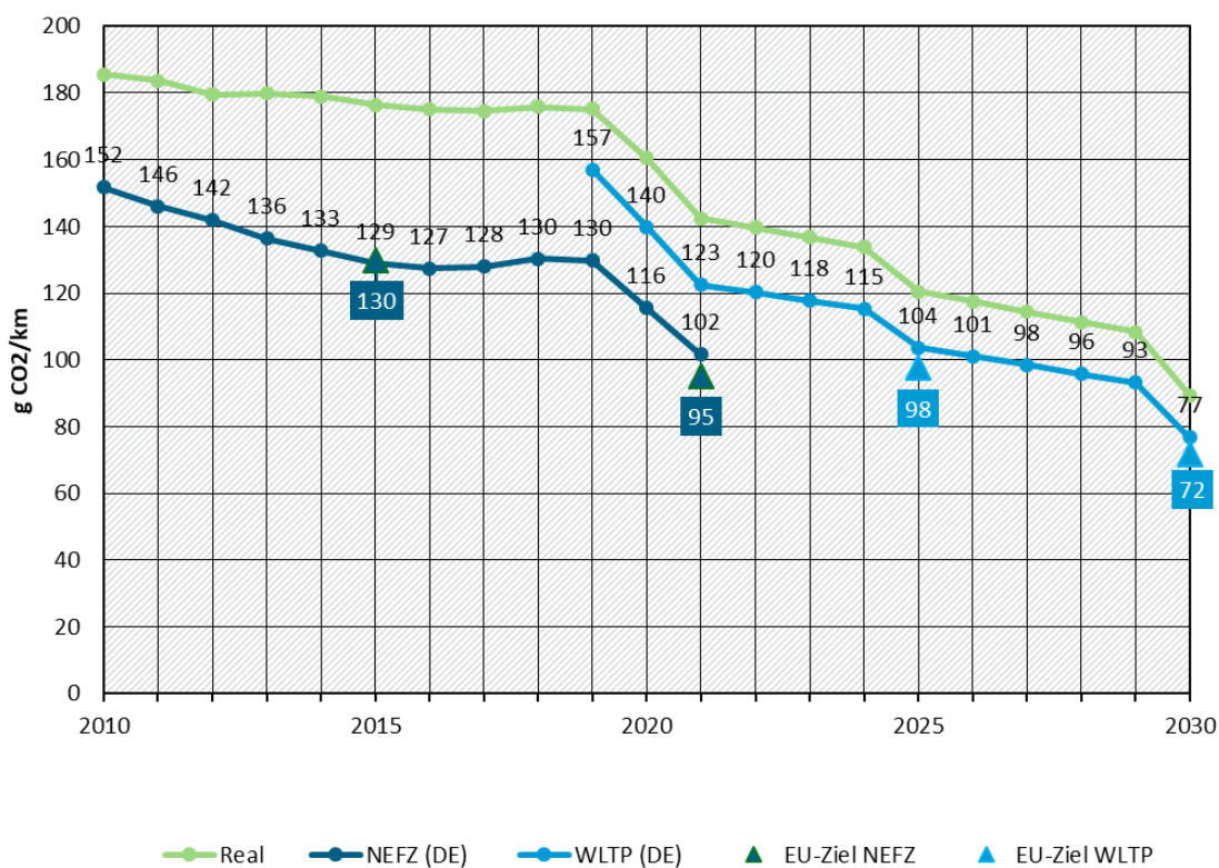
Abbildung 36: CO 2 -Emissionen neu zugelassener Pkw, 2010-2030
