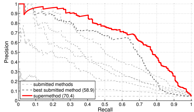
(b) pottedplant
