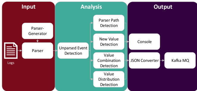
Fig. 4. ÆCID pipeline.
