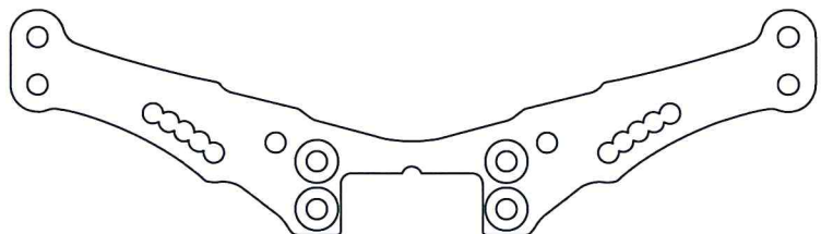
Rear Shock Tower (1) リアショックタワー (1)
