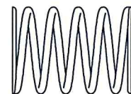
M1.5 x 15 x 25mm 6.75T Spring (4) M1.5 x 15 x 25mm 6.75T スプリング (4)
