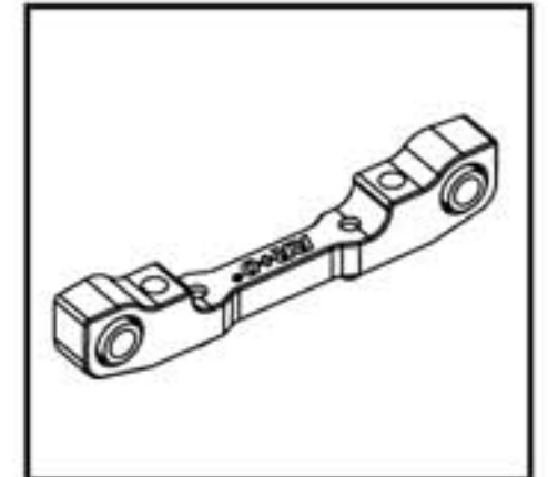
FGX-317/PK Aluminium Suspension Mount RR-0 アルミサスマウント(RR-0度)
