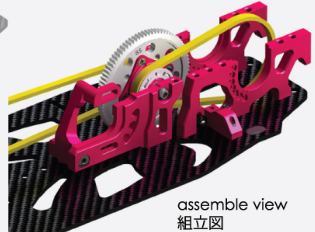
M3 x 8 Button Screw ボタンスクリュー
