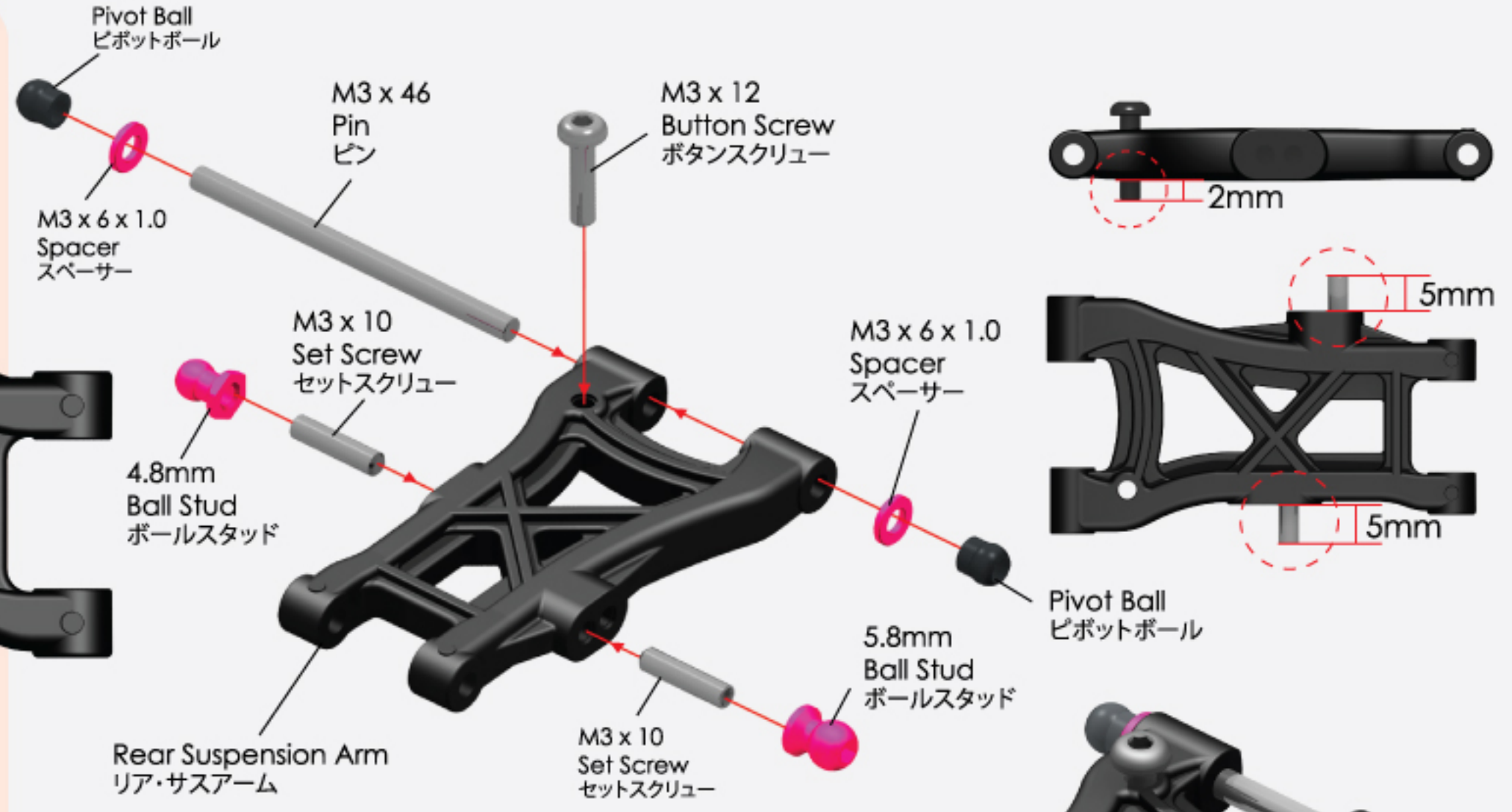
Rear Suspension Arm (2) リア・サスアーム (2)
