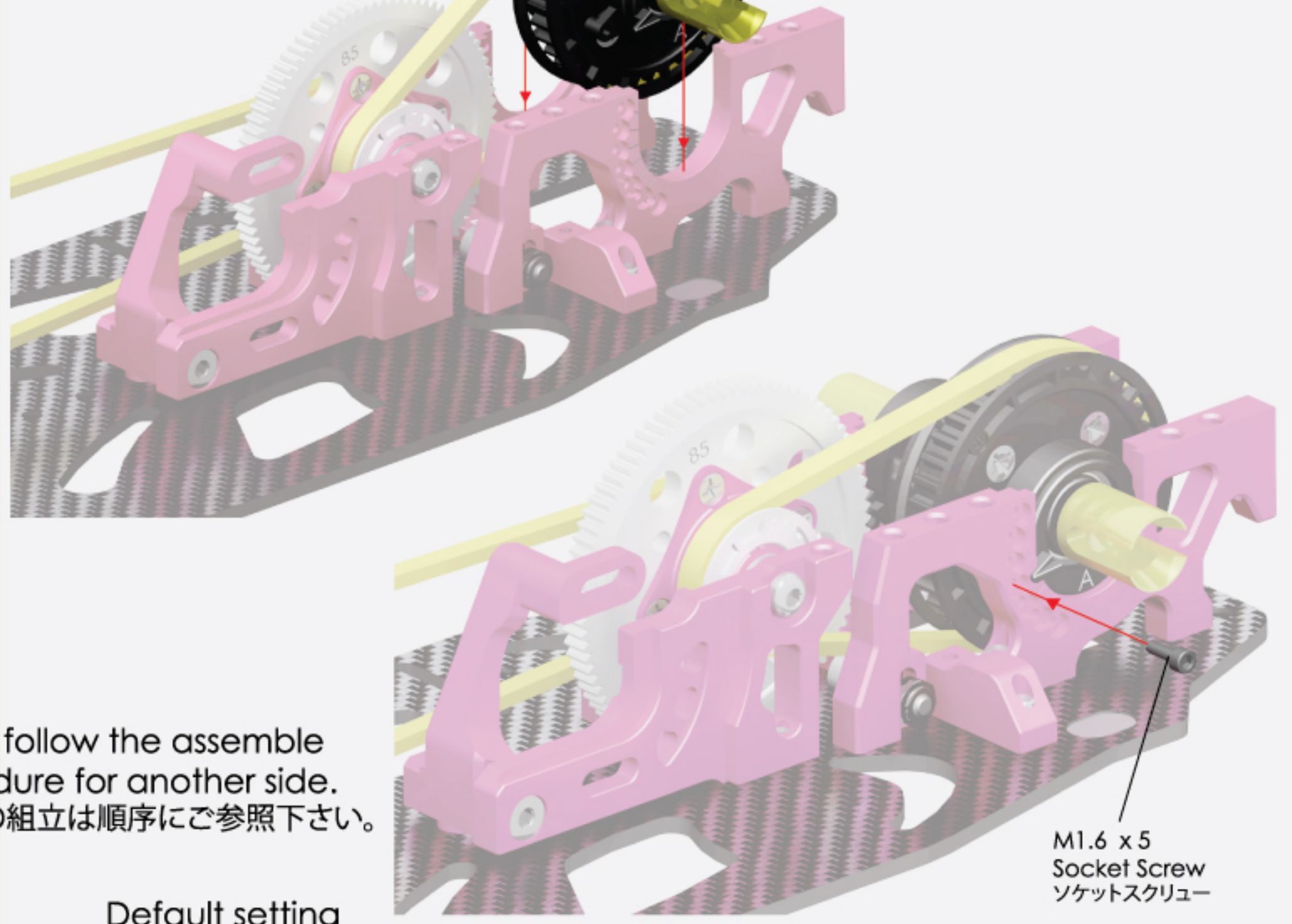
M1.6 x 5 Socket Screw (2) M1.6 x 5 ソケットスクリュー (2)
