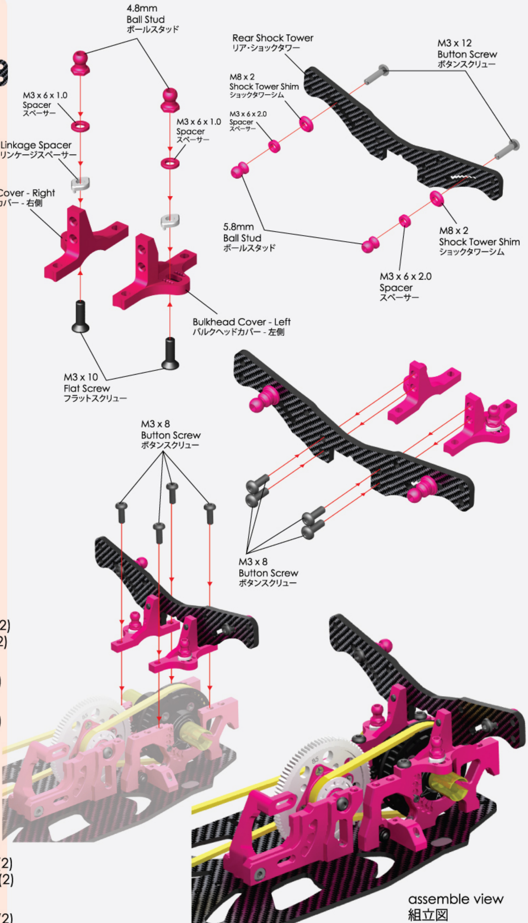
Upper Linkage Spacer (2) アッパーリンケージスペーサー (2)
